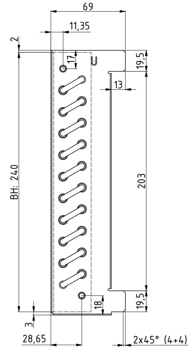
Pohled znázorněn bez ventilátoru View without fan
